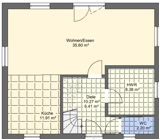
Grundriss Erdgeschoss
