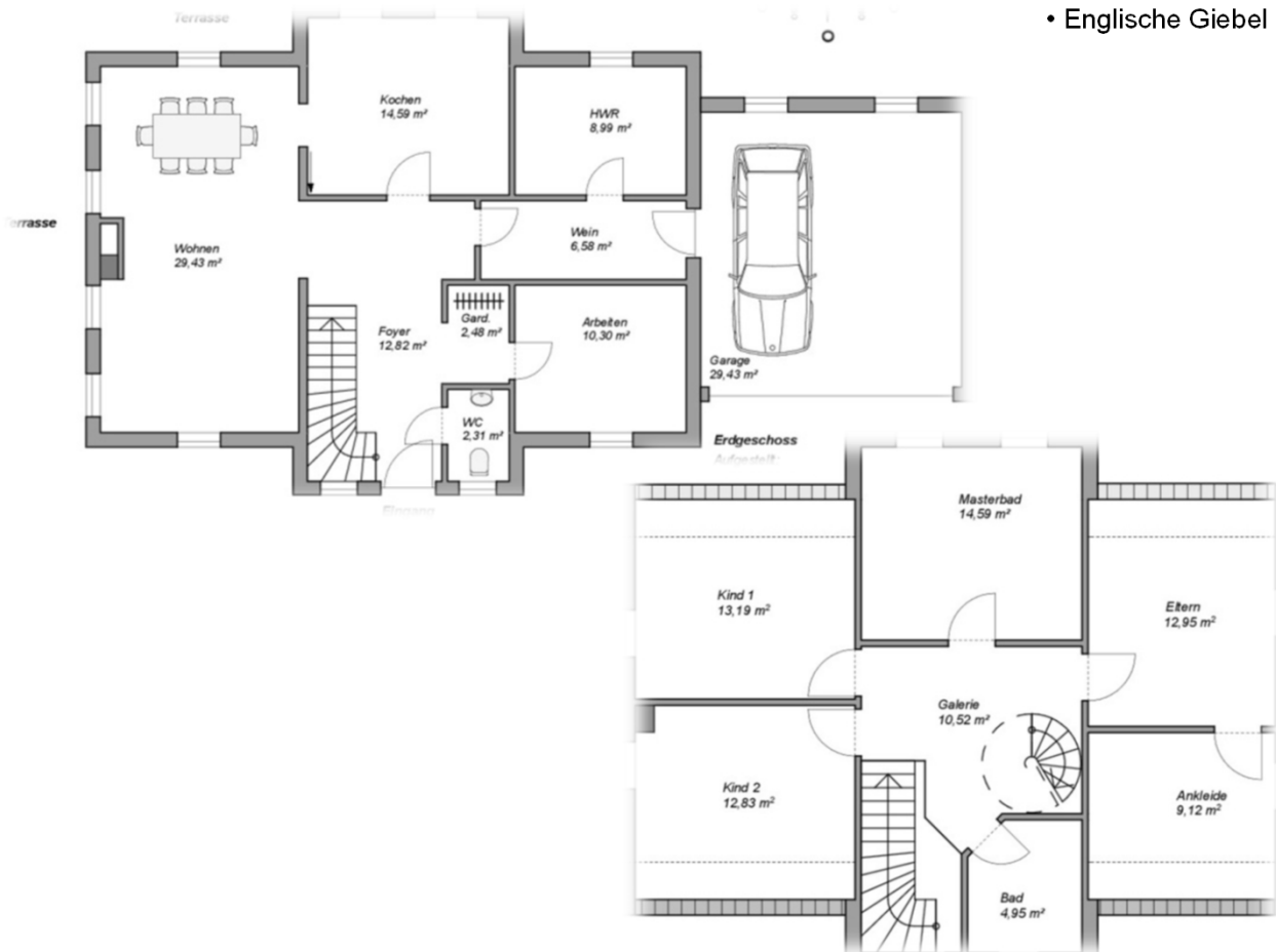
Grundriss Dachgeschoss
